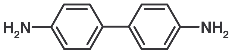
benzidin
